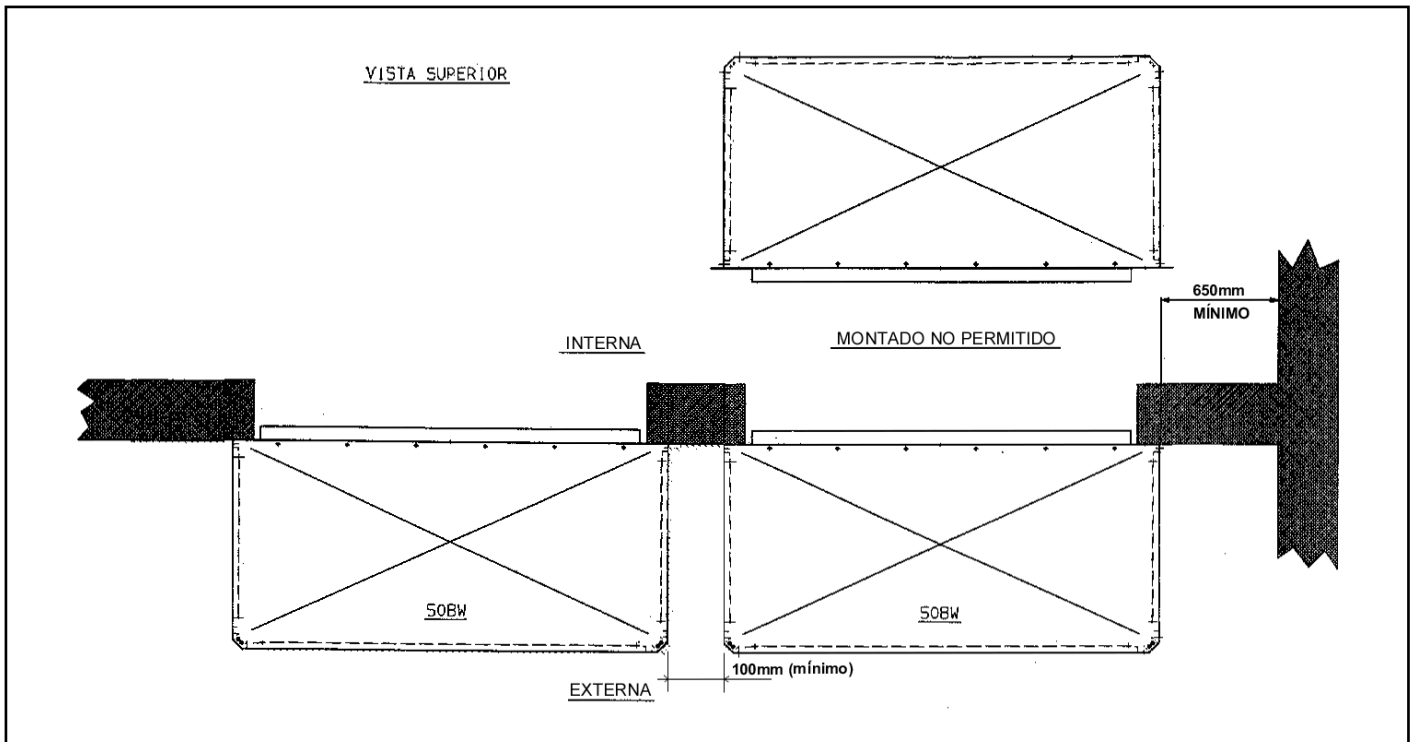
Fig. 5 - Distancias mínimas de montaje
