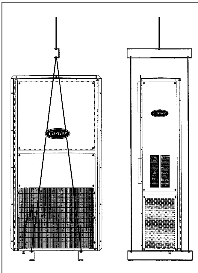
Fig. 1 - Forma de izar
