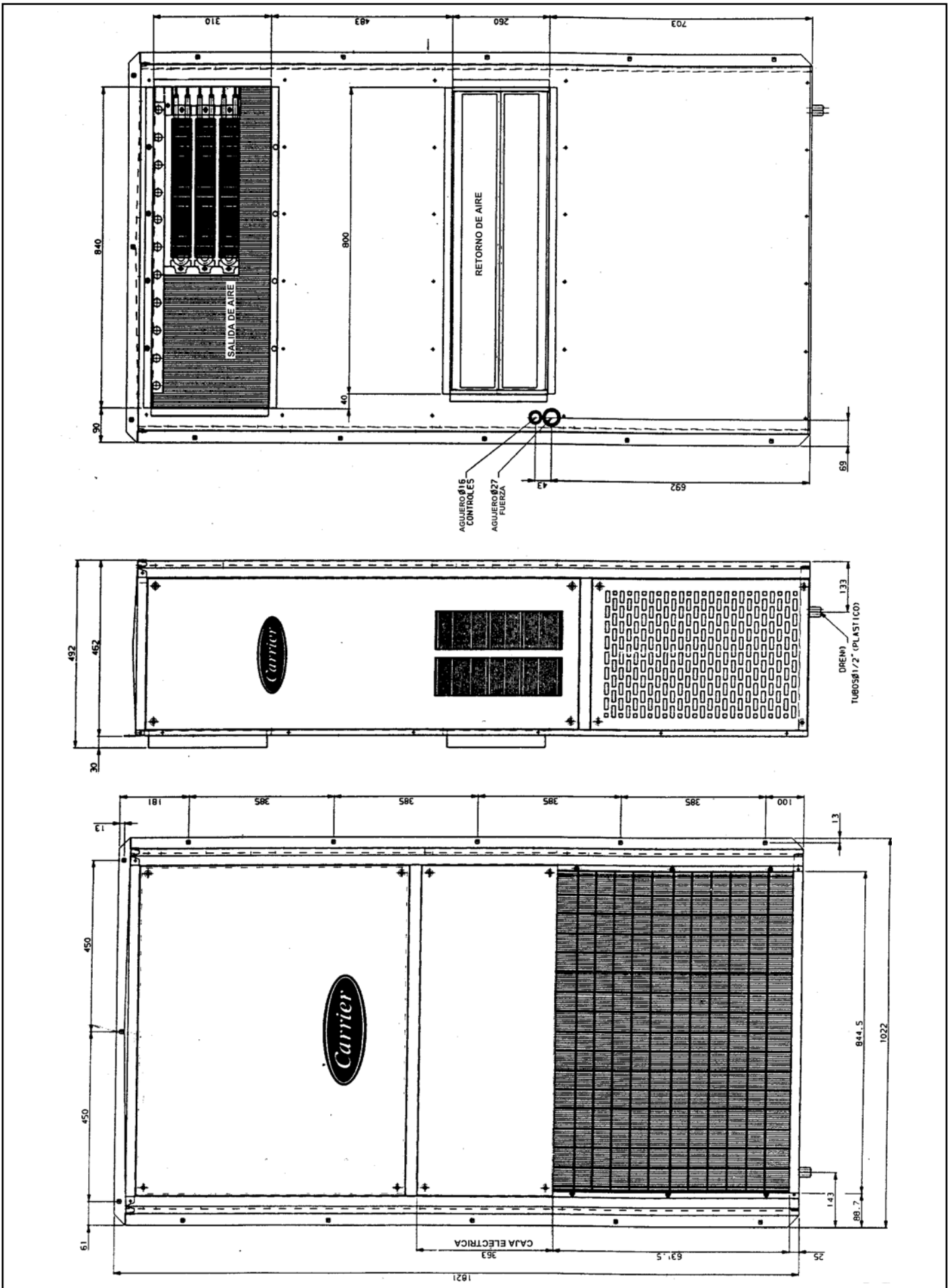
Fig. 2 - Dimensiones de las unidades 50BWA24 / 50BWA36
