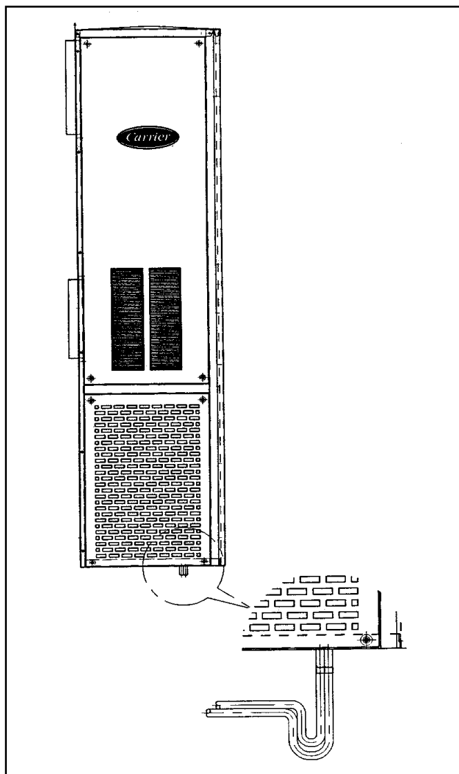
Fig. 6 - Líneas de drenaje
