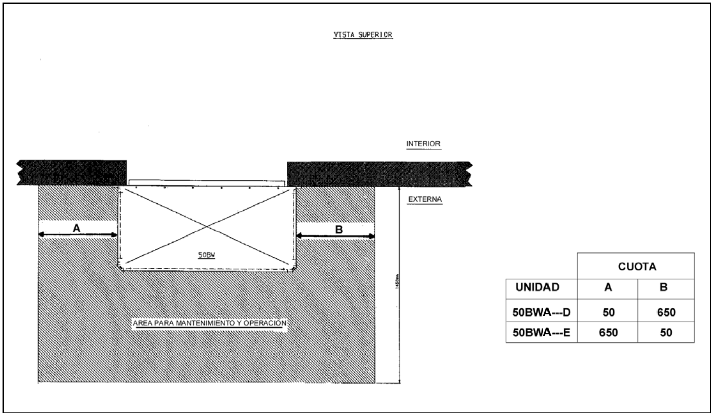
Fig. 4 - Espacios mínimos necesarios para mantenimiento y operación
